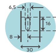
C 4x Montagebohrung
